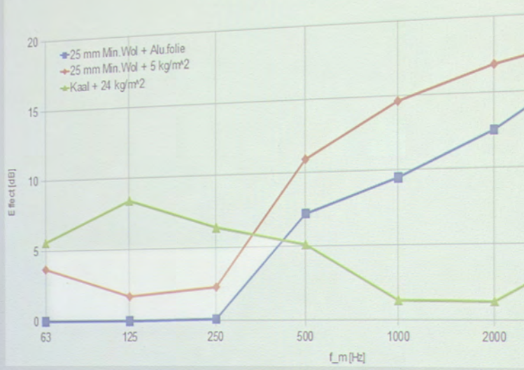
Rechthoekig kanaal 700x300 mm - Effect materialen
